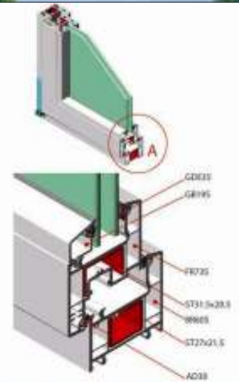
Cửa sổ mở quay vào trong - Cửa sổ mở quay lật vào trong
